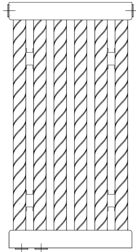
Размеры для подключения "бинокль" 150
