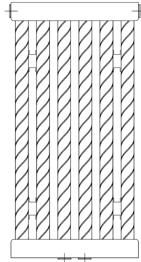
Размеры для подключения "бинокль" 050 по центру
